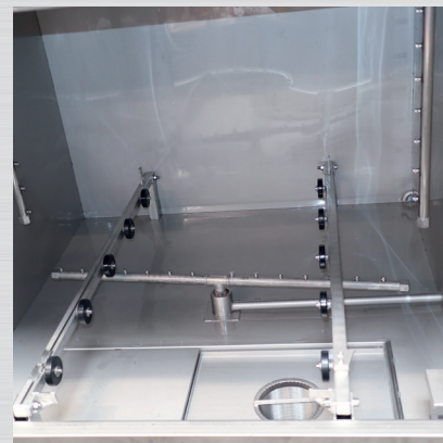
Roterende dysebom fra oven og roterende dyserør fra neden.
